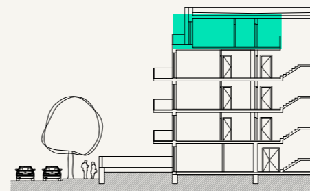
ŘEZ OBJEKTEM
