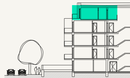
ŘEZ OBJEKTEM
