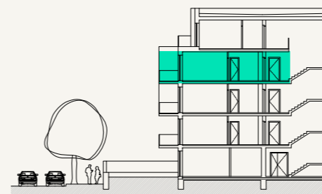
ŘEZ OBJEKTEM
